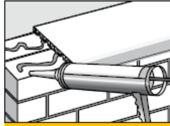
A. gluing
